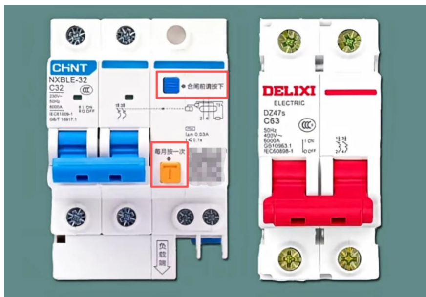
左为漏电保护开关，右为空气开关
